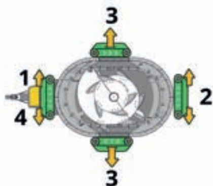
Seria S – konfiguracje taśm wyładowczych
